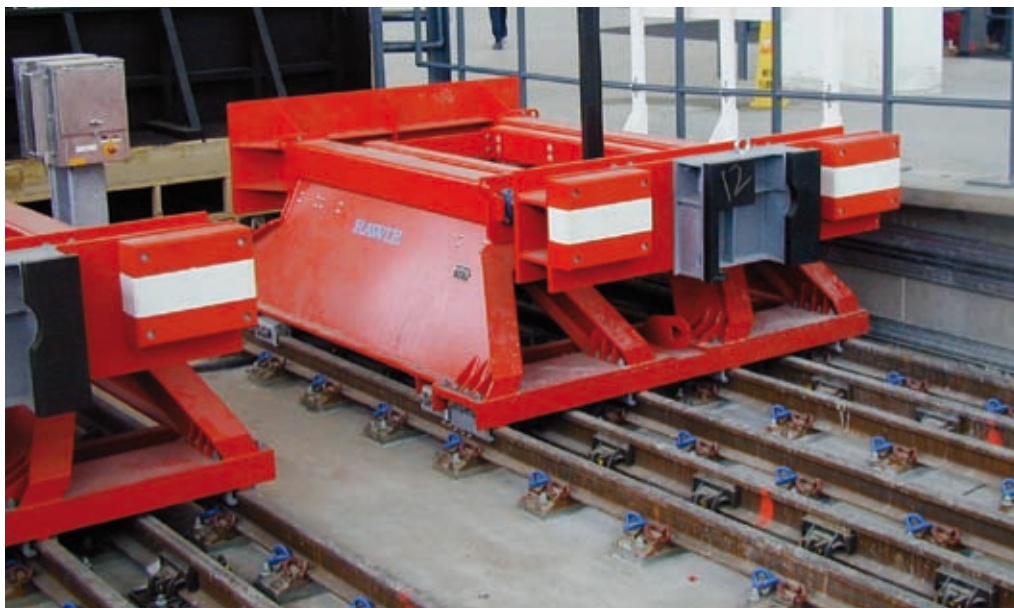
Typ 4 ZEB/14a, Einbauort: St. Pancras Station, London, Großbritannien
